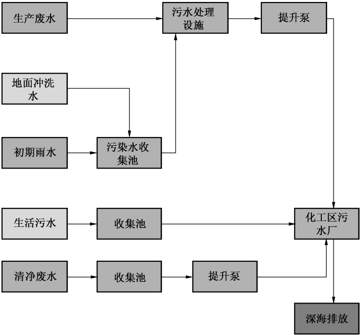
图 A. 24 废水分类示意图
