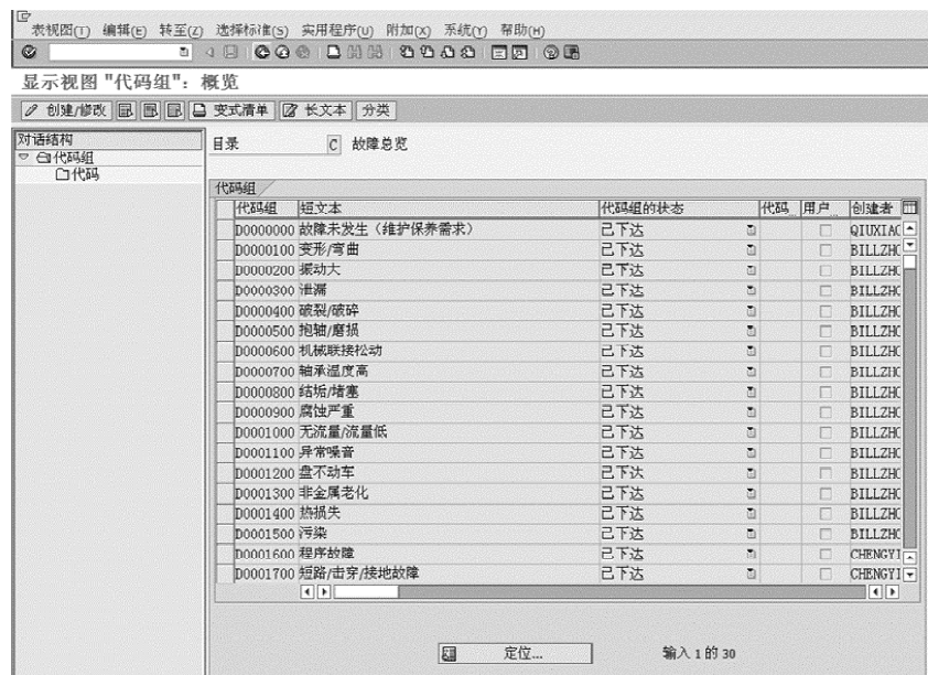
图 A.14 SAP 中失效模式的统计
