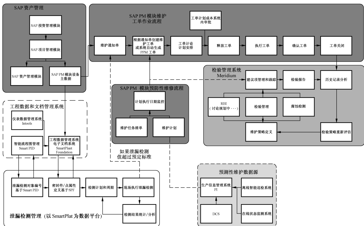
图 A.12 设备维护系统模块图
