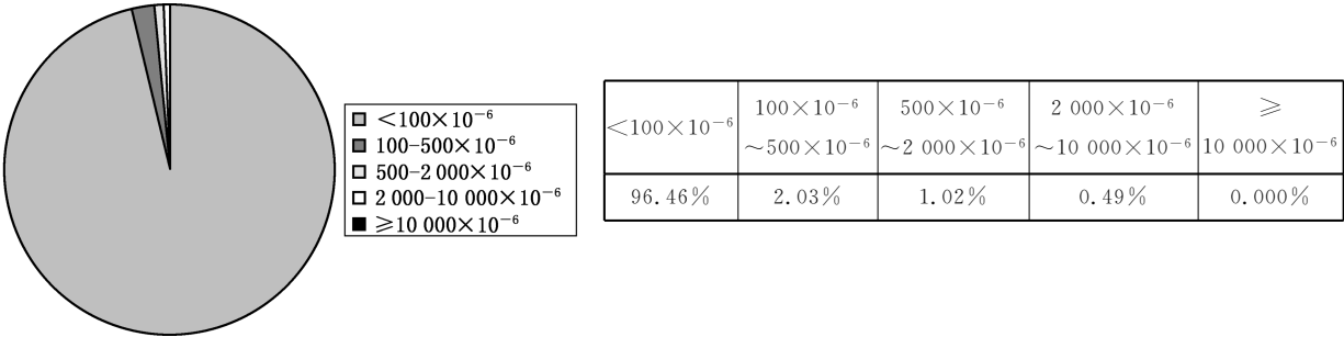
图 A. 17 泄漏检测数据
