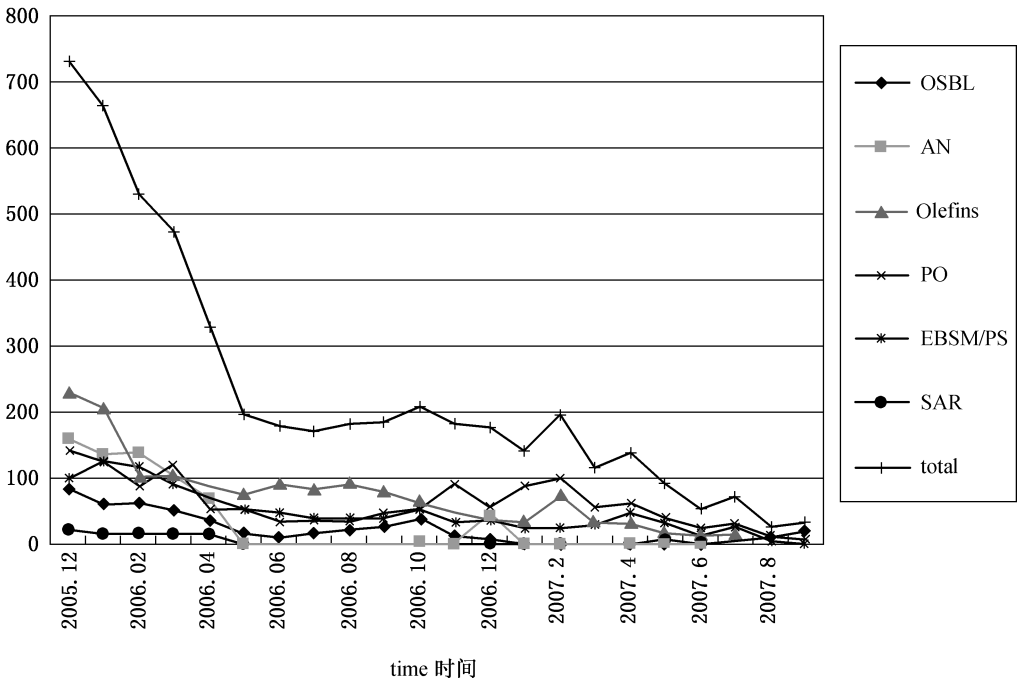
图 A. 18 安全阀过期趋势
