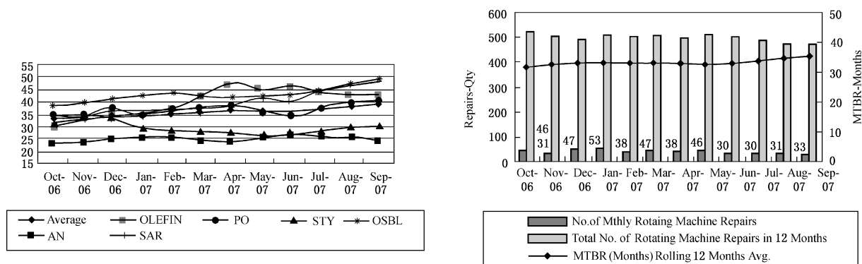
图 A.15 动设备平均维修间隔时间
