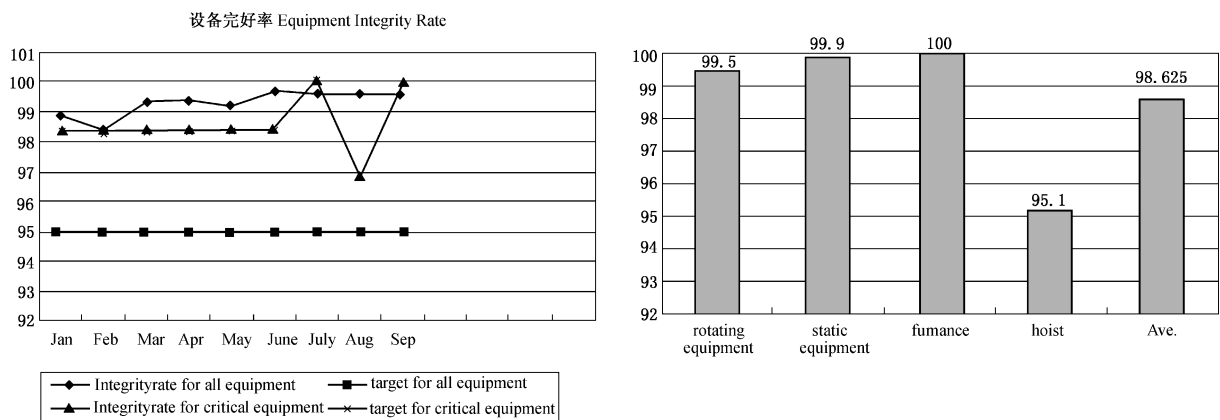
图 A.16 设备完好率
