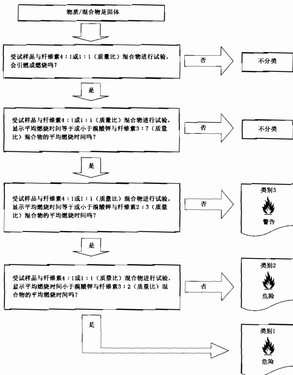
图 1 氧化性固体判定流程
