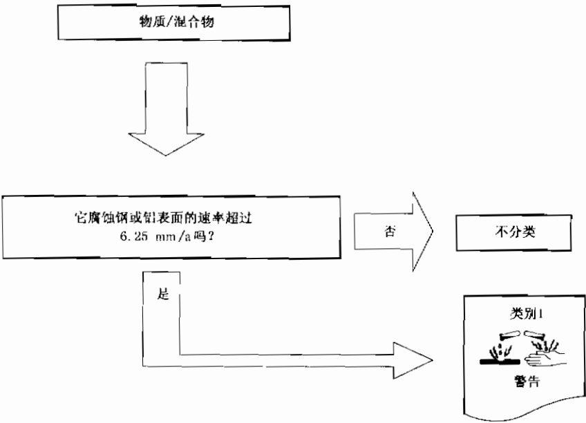
图 1 金属腐蚀物质和混合物的判定流程
