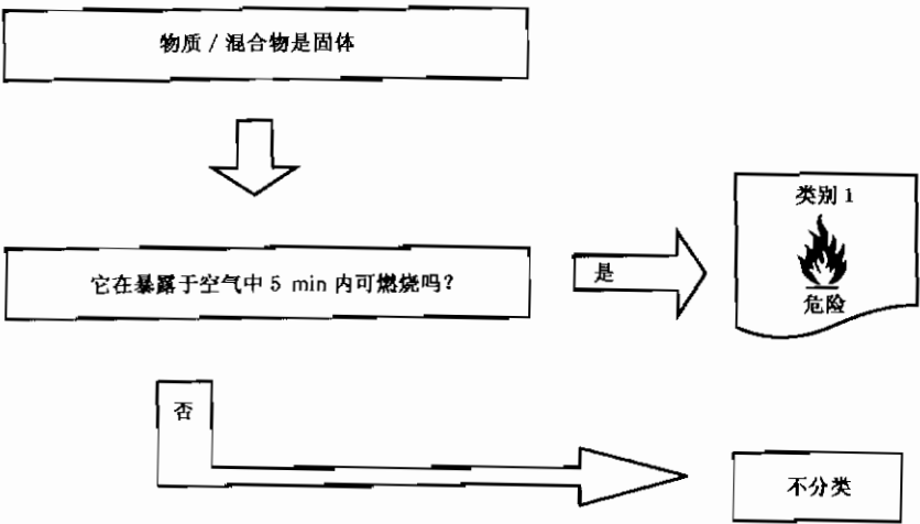
图 1 自燃固体判定流程
