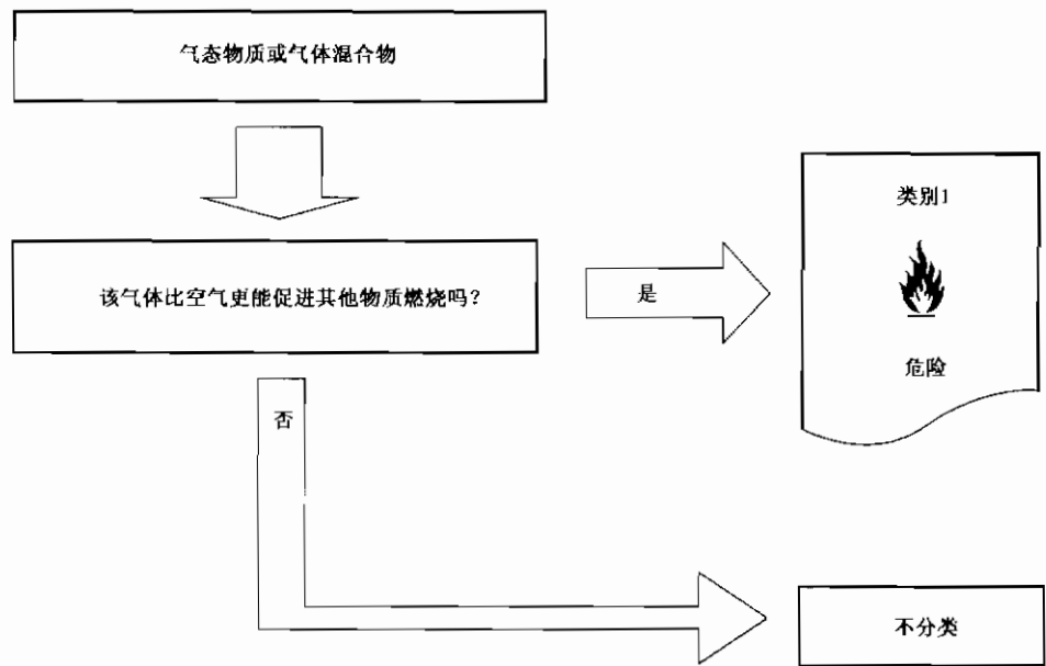
图 1 氧化性气体判定流程
